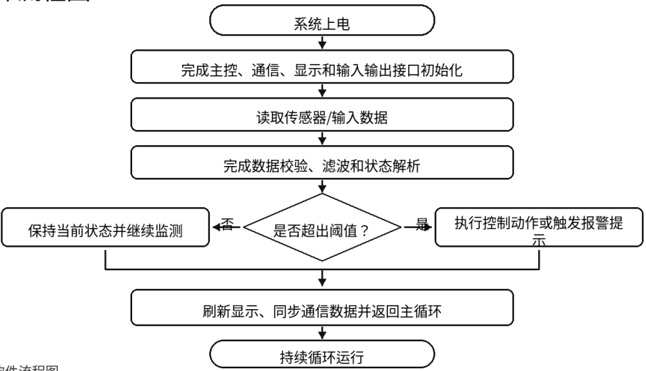
图2 软件流程图
